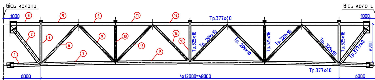
Рис. 1. Ферма підкроквяна ПФ-6
