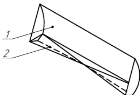
Рис. 6. Відвал з комбінованою ножовою системою
